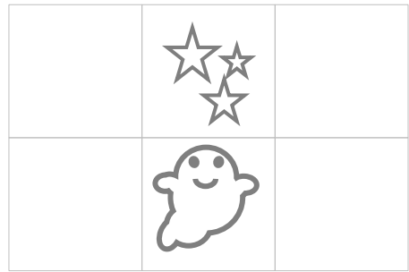
プログラム 2
