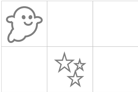
プログラム 3
